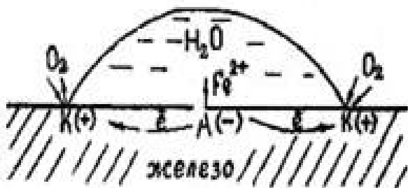
Рис. Коррозия при неравномерной аэрации
